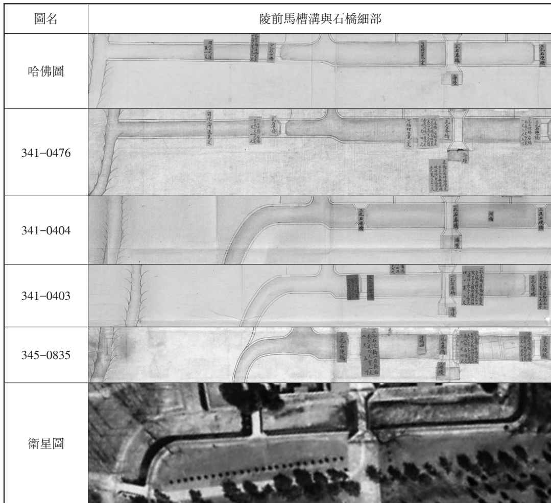
圖7 陵前馬槽溝與石橋細部對比圖
