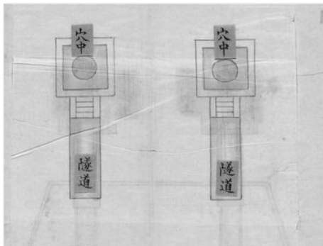
圖2 繪製在宣紙上的寶頂平面圖
